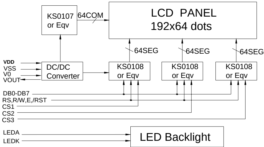
19264 点阵系列 3 片选模块原理框图
