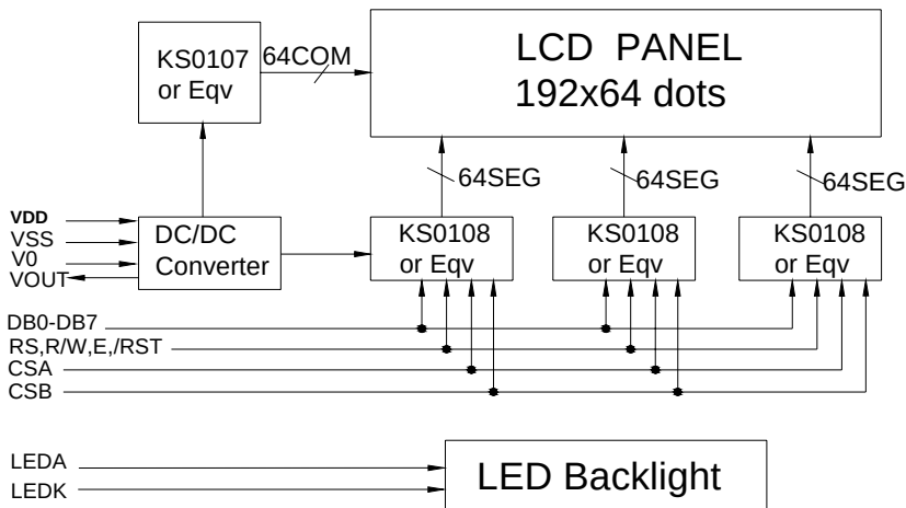
19264 点阵系列 2 片选模块原理框图
